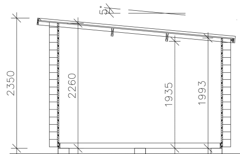
Sektion
