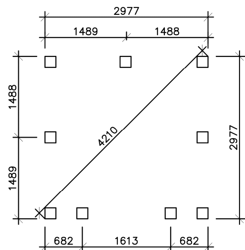
Plintritning
