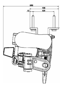
Takmontage
