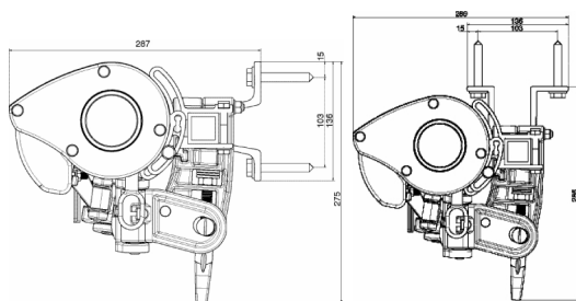
Semi väggmontage
