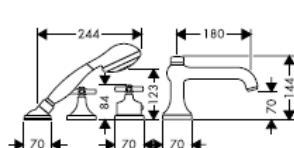
Terrano 37461XXX
