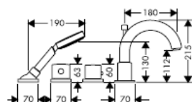
Uno 38461XXX
