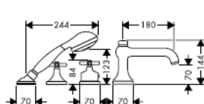
Terrano 37461XXX
