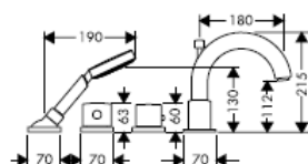
Uno 38461XXX
