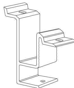
Takstolskonsol 27°
