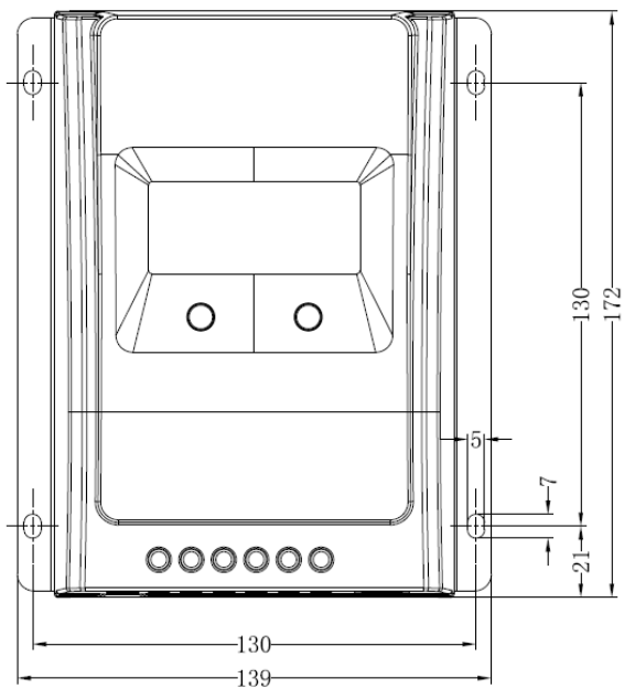
Tracer3210A Dimensioner i millimeter
