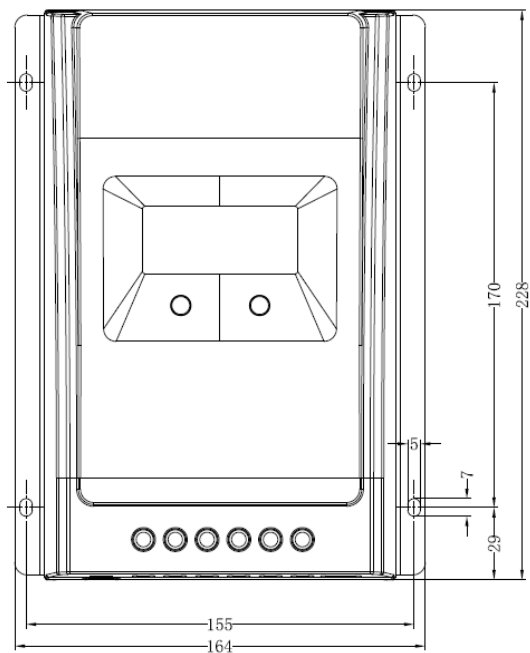
Tracer4210A Dimensioner i millimeter
