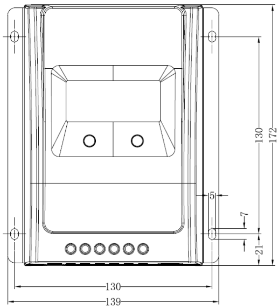
Tracer2210A Dimensioner i millimeter
