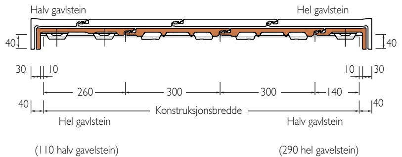
Bruk av gavlstien for Zanda Minster.
