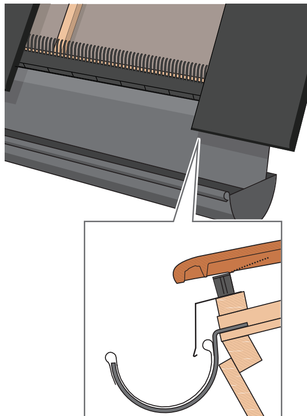
Ved bruk av flat takstein skal det benyttes ventilert fuglelist.
