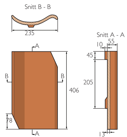
DANTEGL
