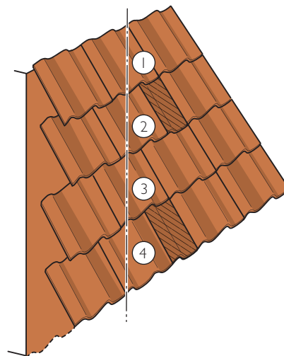
Forskyv kappelinjen til den samme vinkelen, slik at steinen ikke blir mindre enn halv, se tegning.
