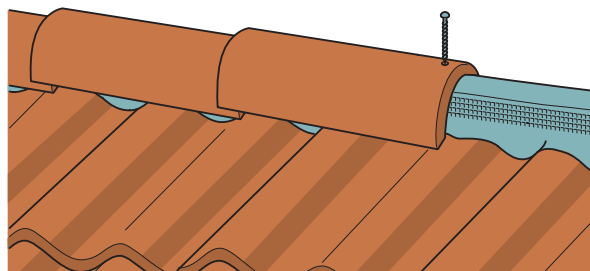
Feste møne- og valmstein med skruer m/pakning eller spiker m/pakning.
