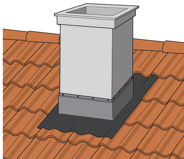
Tette skorsteinen med Wakaflex.
