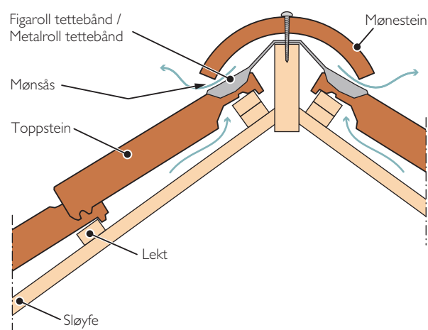
Møneløsning.
