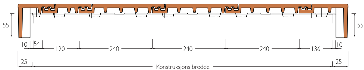
Turmalin med gavlstein.
