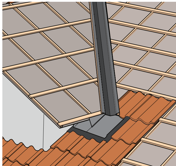
Vinkelrenne skuff.
