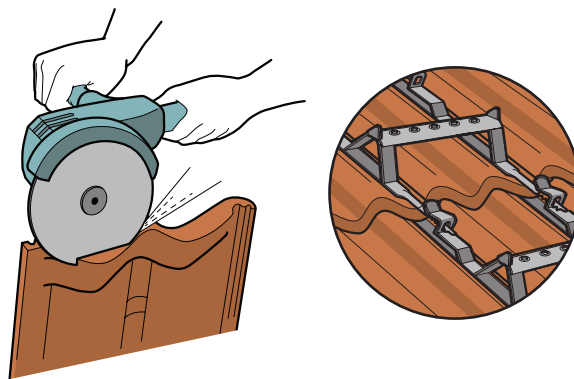
Gjennomføringer i overlappen gjøres for å unngå punktbelastninger og for å ivareta tettefunksjonen.
