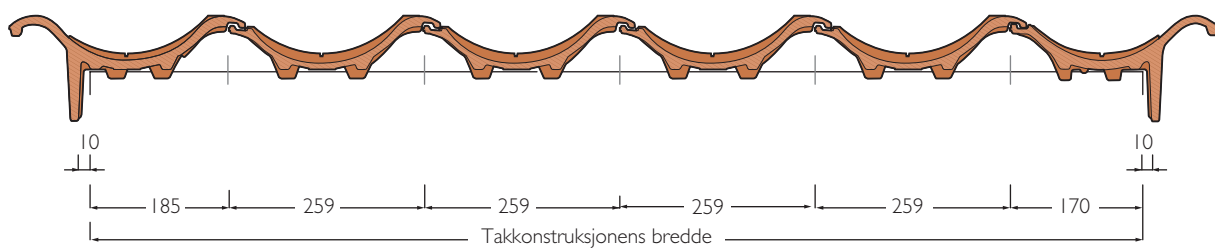
Nortegl med gavlstien.
