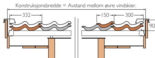
Konstruksjonsbredde uten bruk av gavlstein for Zanda betongtakstein..
