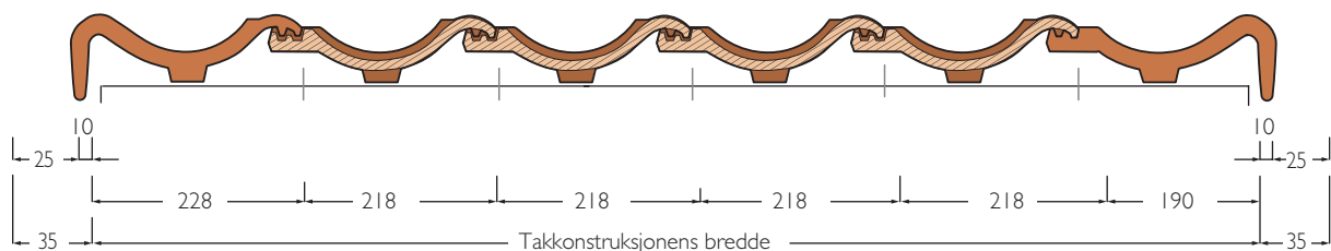
KDN VH med gavlstien.
