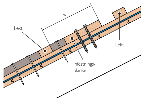
Innfestningsplanke.
