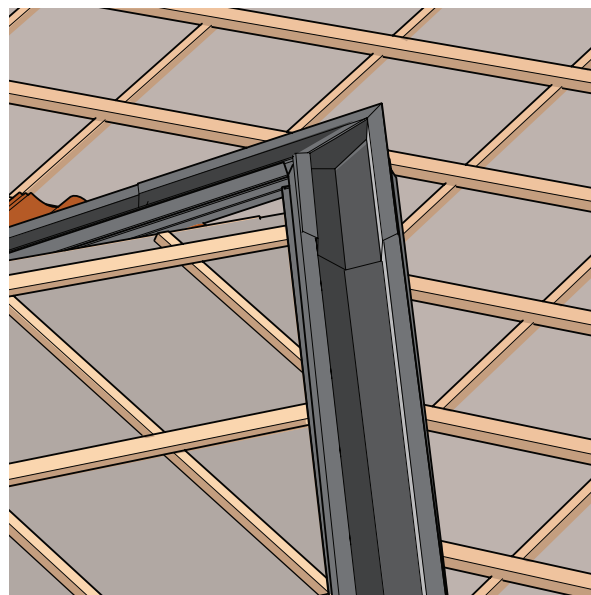
Vinkelrenne topp.
