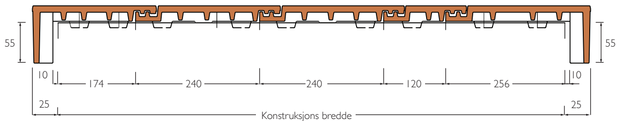
Med halv gavlstein
