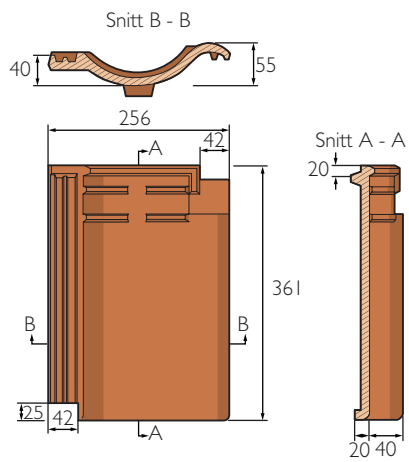
KDH VH
