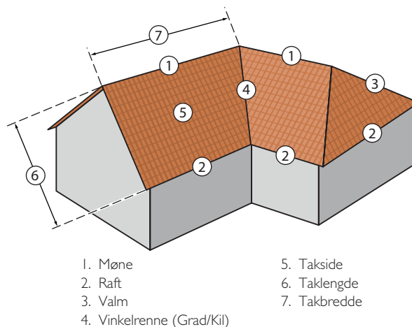
Betegnelser på takdeler.
