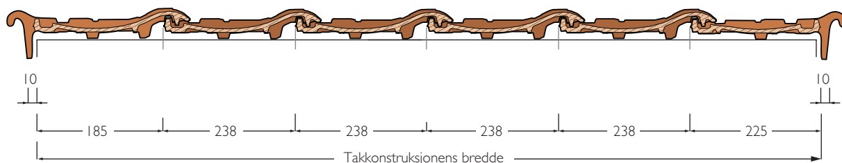
Nova med gavlstien.
