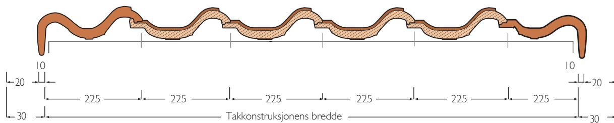
Hollander med gavlstien.
