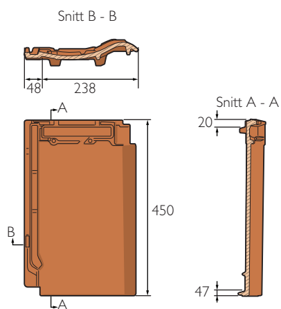
NOVA
