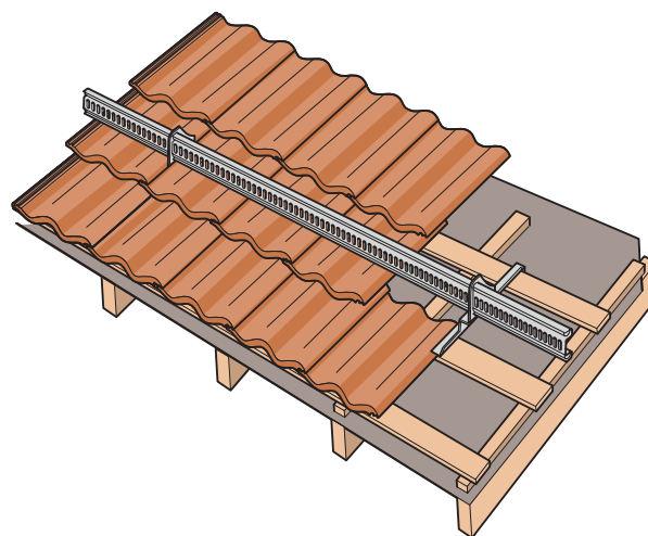
Snøfangere.
