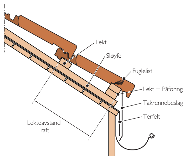
Opplekting ved raft.
