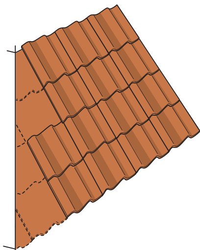
Legg så mange hele steiner som mulig uten at de overlapper vinkelrennen eller valmmønnet, se tegning.
