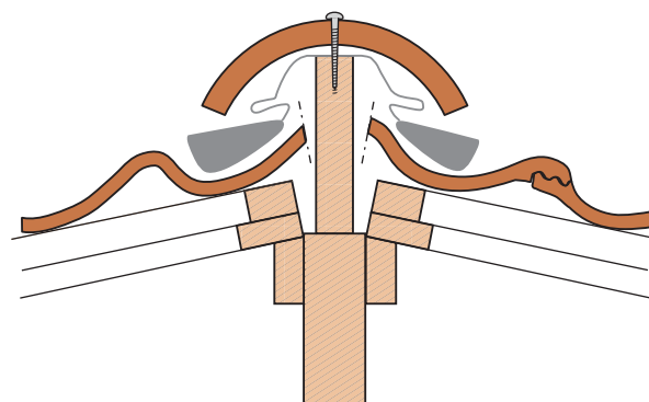
Metalroll tettebånd.
