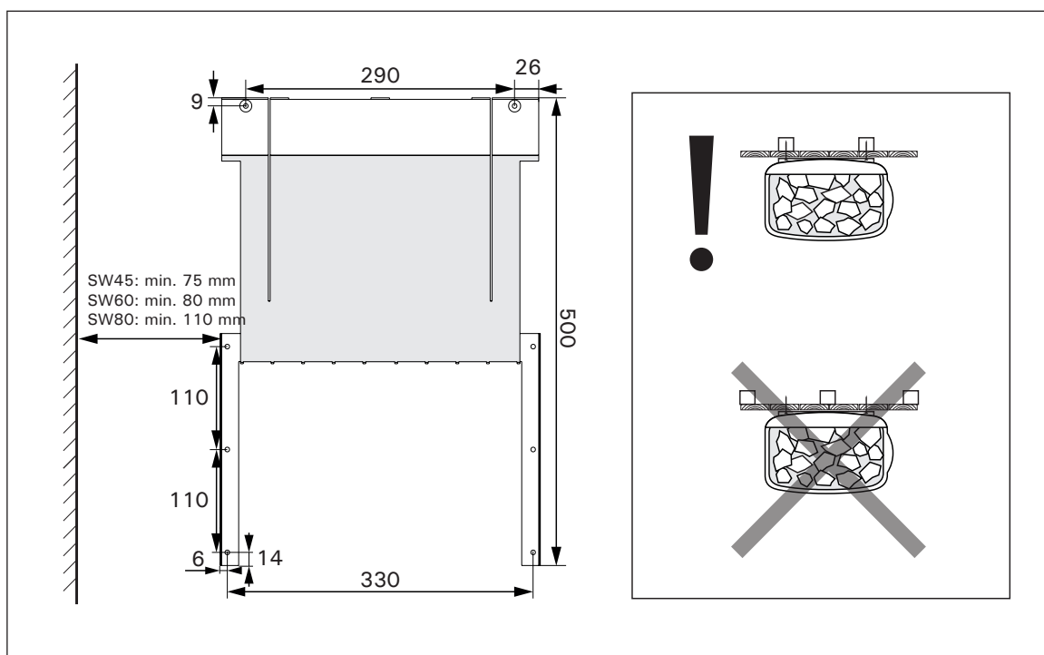
Kuva 6. Seinäteline, mitat millimetreinä Bild 6. Vägkonsolen, måtten i millimeter
