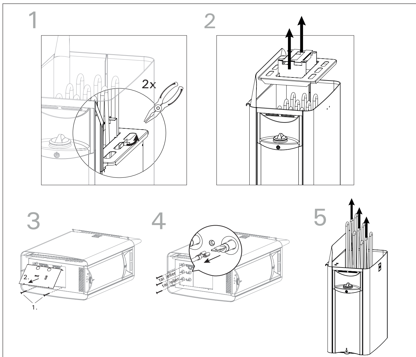
Kuva 9. Vastusten vaihtaminen Bild 9. Byte av element
