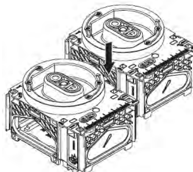
Kopplingsschema
