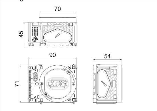
Måttritning
